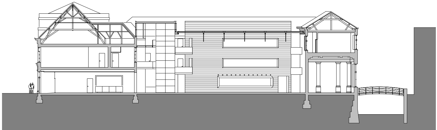
Langsdoorsnede Jeroen Boschhuis, atrium, trommel, pleitzaal en brug over de Binnendieze
