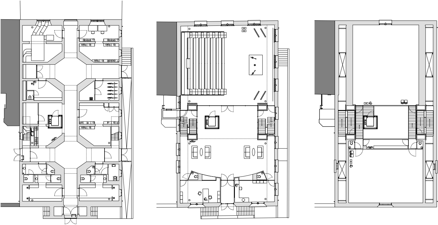
Plattegronden souterrain, begane grond en eerste verdieping
