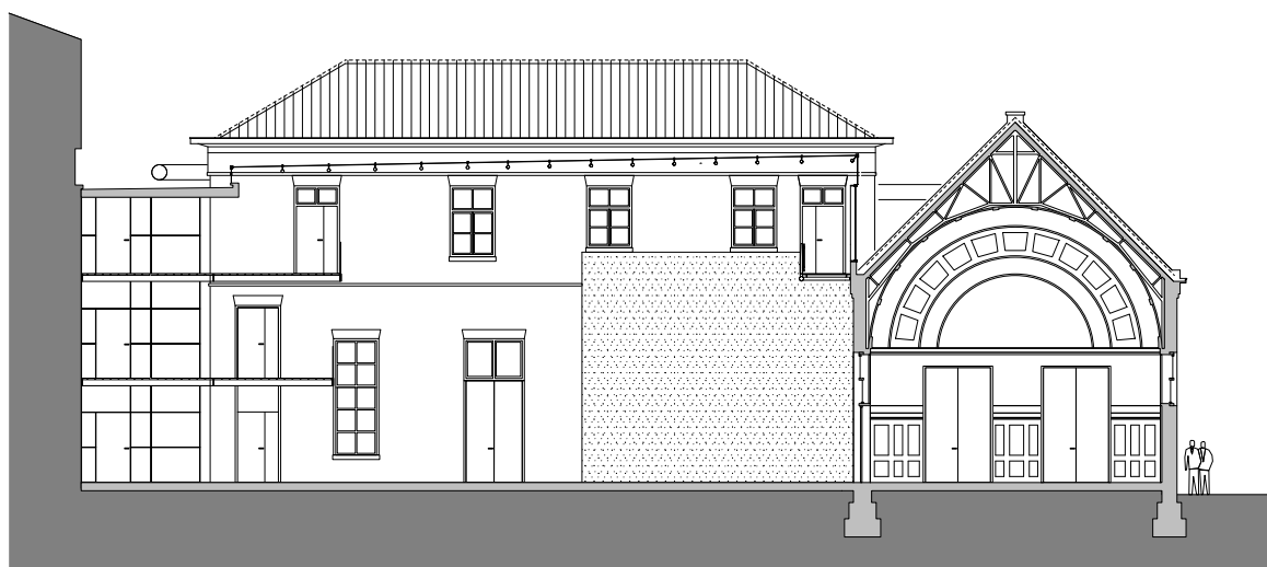
Dwarsdoorsnede overloop, atrium en pleitzaal
