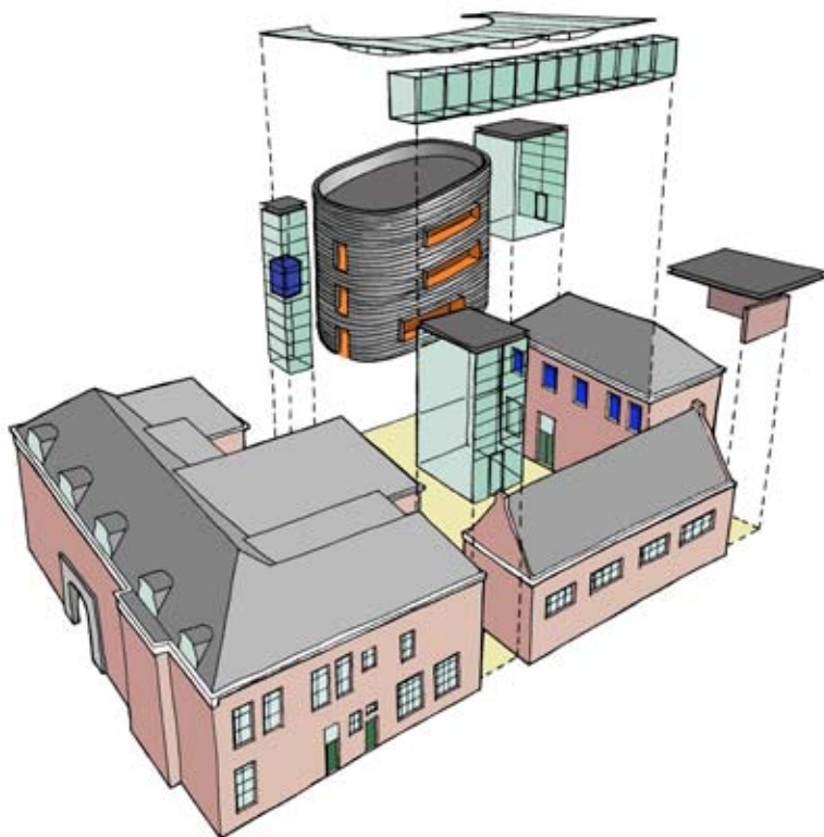
Exploded view nieuwe toevoegingen
