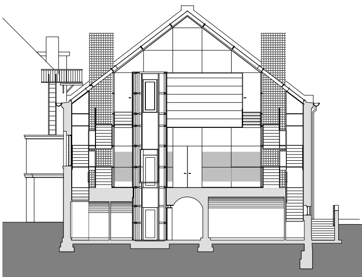
Boven: dansstudio Onder: dwarsdoorsnede en trappenhuis
