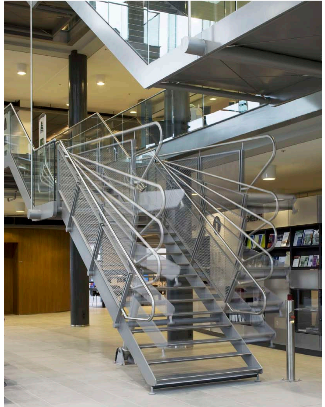
Een elektrisch te bedienen trap sluit de bibliotheek als een ophaalbrug af van de entree hall. The electrical stairs close the library like a drawbridge from the entrance hall.
